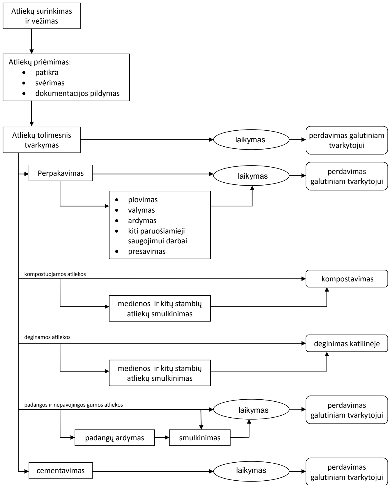
1 pav. Technologinių procesų principinė schema
