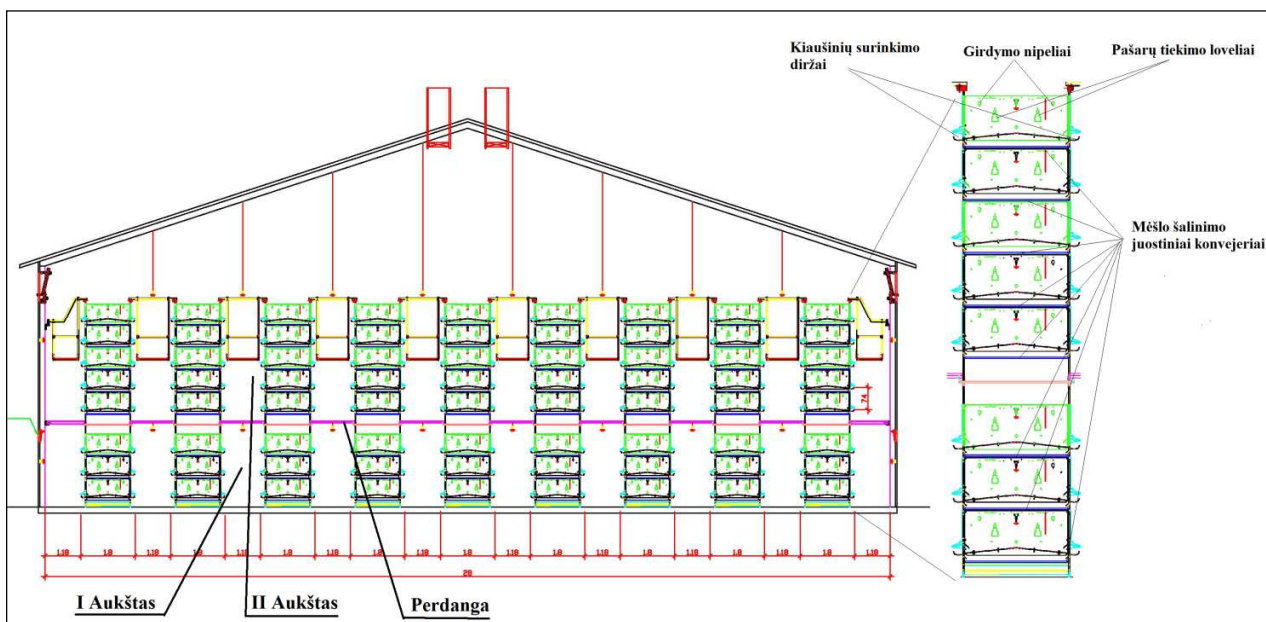
7 pav. Vištų laikymo narvų išdėstymo vištūdeje pavyzdys.
