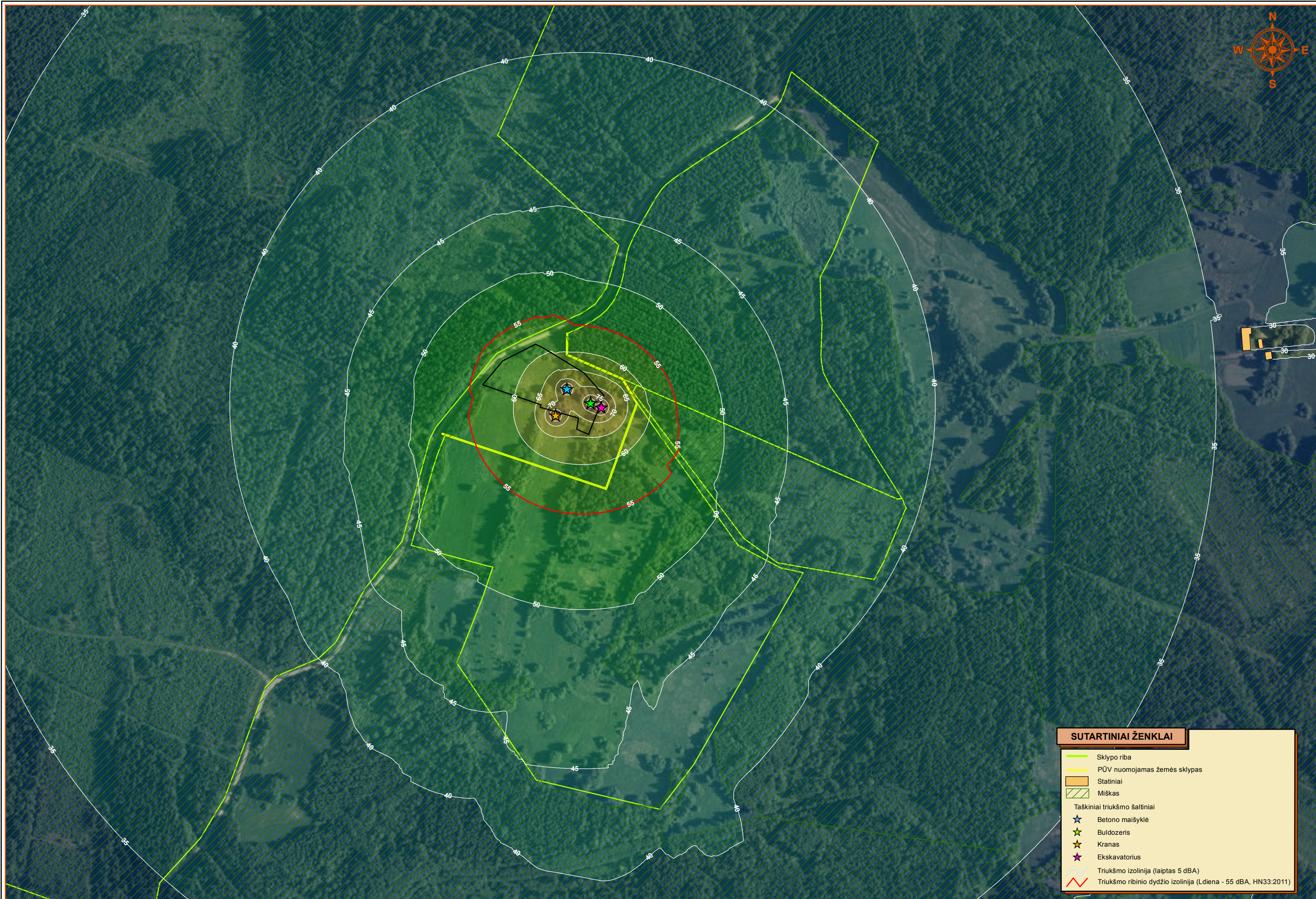
Naftos gavybos aikštelės įrengimo metu įrangos sukeliama akustinio triukšmo sklaidos matematinio modeliavimo Pyvorų NGA aplinkoje rezultatų schema (Ldiena)
