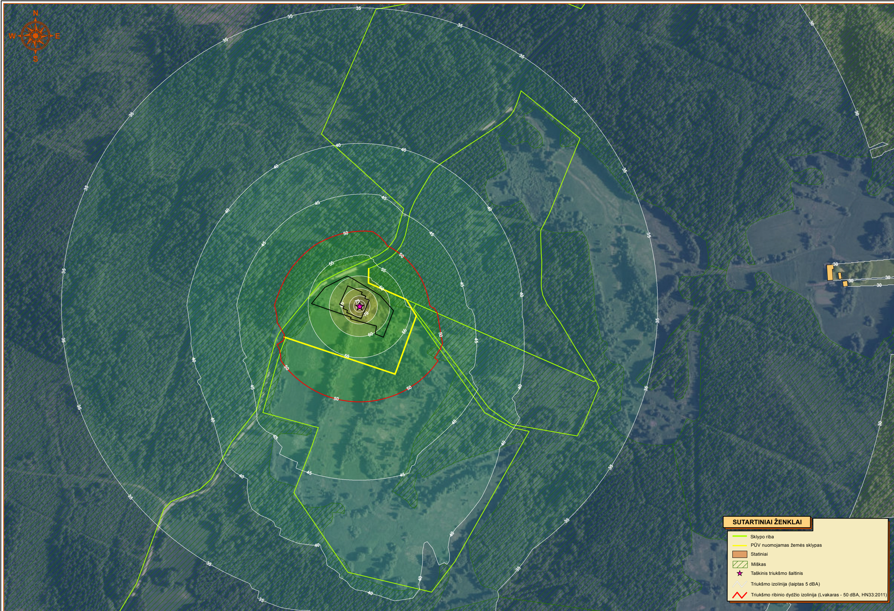
Gręžinio gręžimo metu sukeliama akustinio triukšmo sklaidos matematinio modeliavimo Pyvorų NGA aplinkoje rezultatų schema (Lvakaras)
