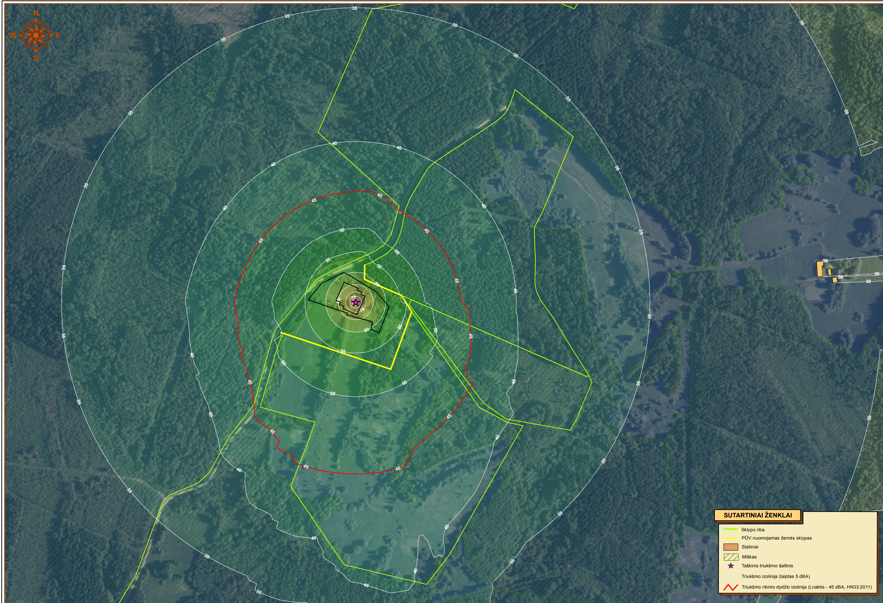
Gręžinio gręžimo metu sukeliama akustinio triukšmo sklaidos matematinio modeliavimo Pyvorų NGA aplinkoje rezultatų schema (Lnaktis)
