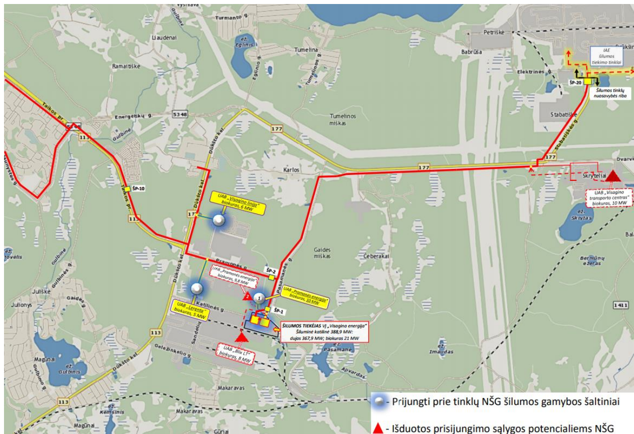
Pav. 4. Prie VI „Visagino energija“ šilumos perdavimo tinklų prijungti ir planuojami prijungti nepriklausomų šilumos gamintojų (NŠG) šilumos gamybos šaltiniai
