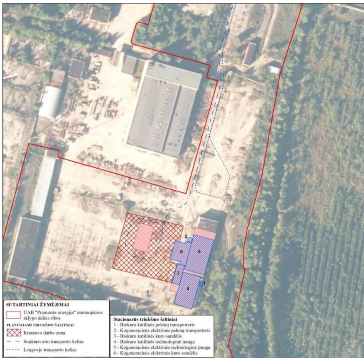
Pav. 3. Triukšmo šaltinių schema
