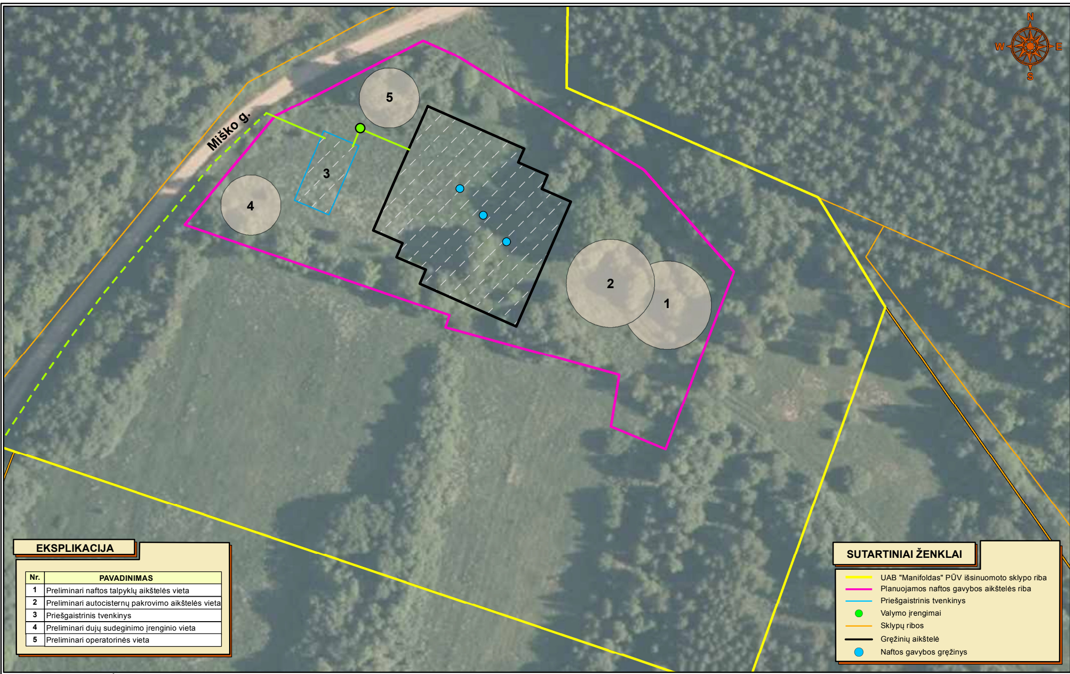
Pyvorų NGA preliminari įrengimų išdėstymo schema
