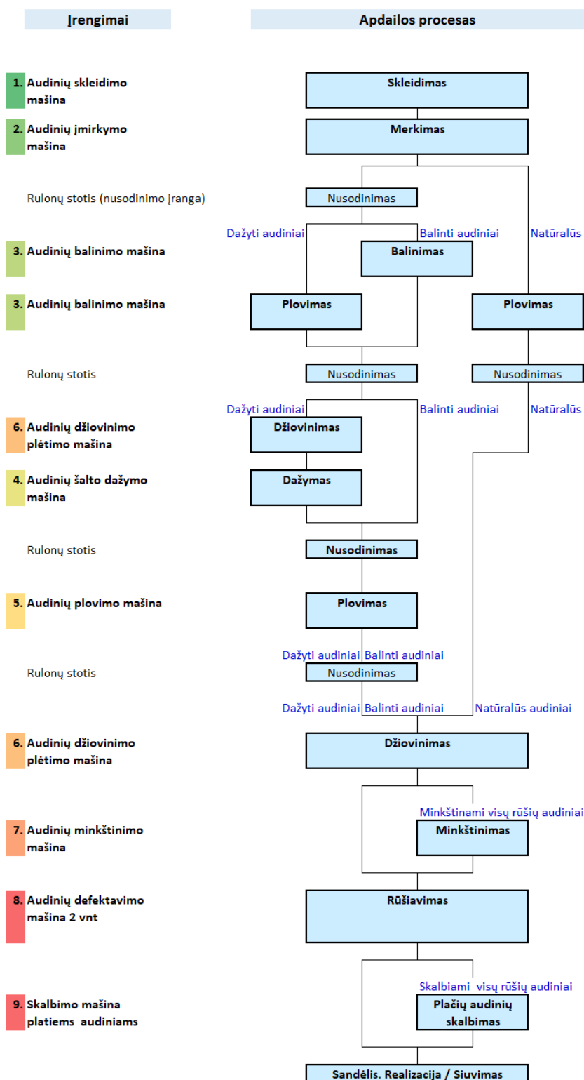
5 pav. Apdailos technologinio proceso schema
