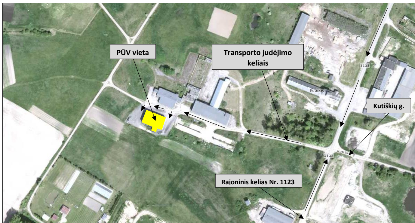
3 pav. Transporto judėjimo maršruto į planuojamos ūkinės veiklos teritoriją schema
