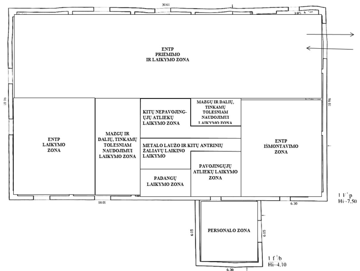
2 pav. Eksploatuoti netinkamų transporto priemonių (ENTP) tvarkymo veiklos patalpų schema
