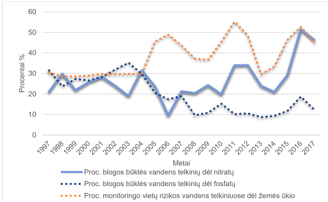
Pav. 7. Valstybinio upių monitoringo tyrimų vietų dalis, kuriose nitratų azoto ir fosfatų fosforo koncentracijos neatitinka „geros“ būklės kriterijų, ir stebėsenos vietų dalis rizikos vandens telkinių baseinuose dėl žemės ūkio poveikio. Čia bloga būklė suprantama kaip bet kokia būklė, kuri neatitinka geros arba labai geros būklės.
