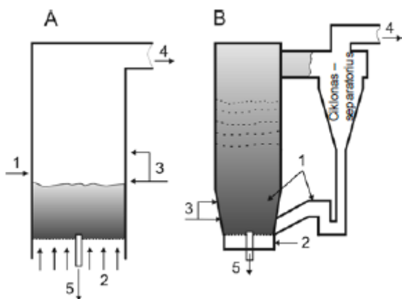
Pav. 2.1.3. Principinė pakuros su stacionariuoju (A) ir cirkuliuojančiuoju (B) verdančiu sluoksniu schema 26
