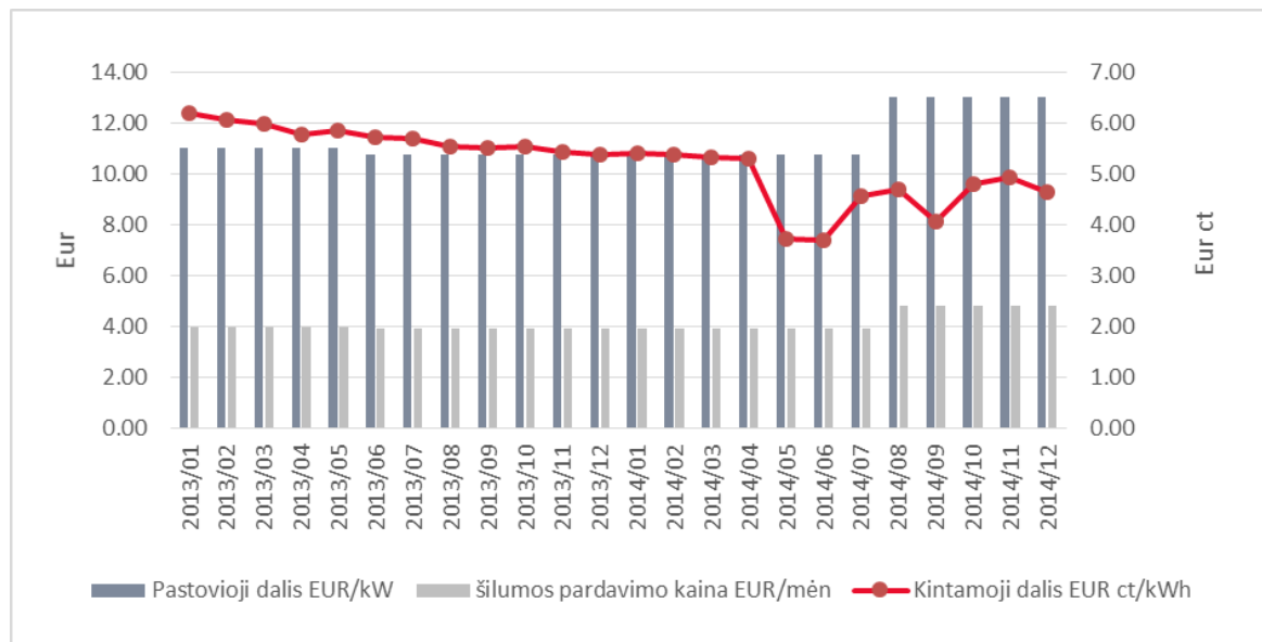
Pav. 4.7.6. Dvinarės šilumos kainos dedamųjų kaita 2013–2014 metais.
