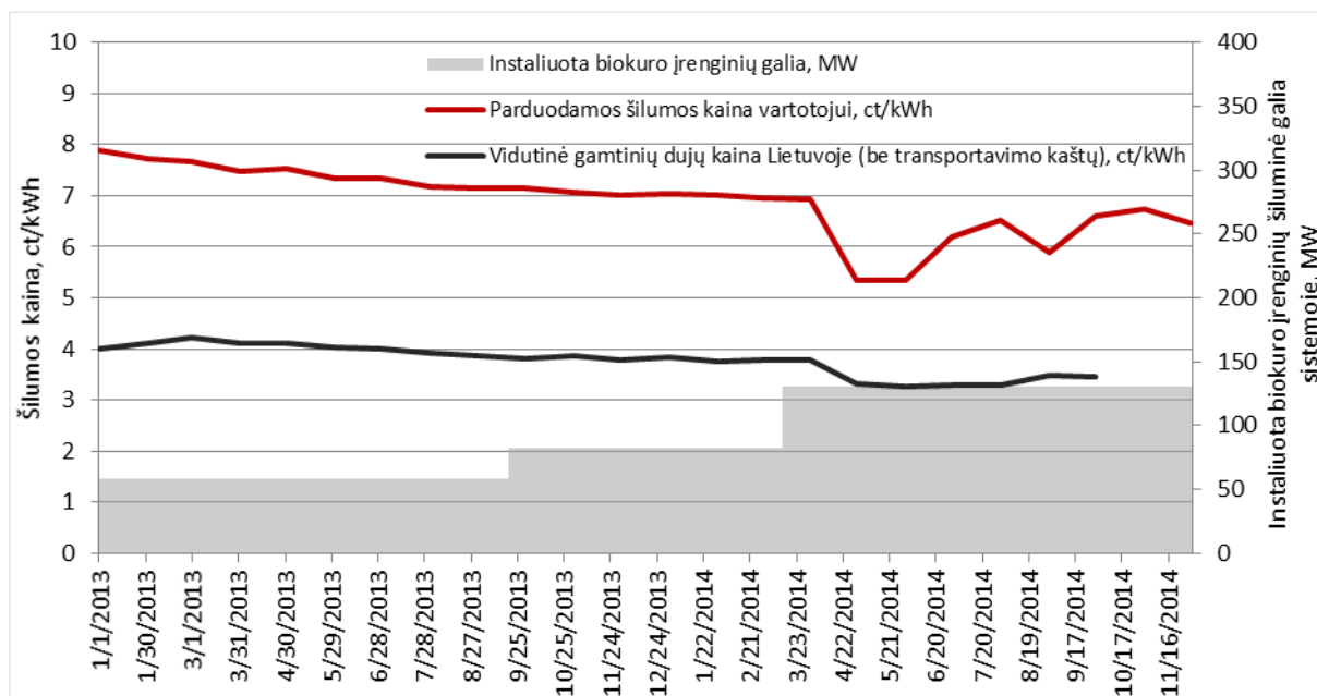
Pav. 4.7.4. Vilniaus IT šilumos energijos kainos priklausomybė nuo instaliuotų biokurą naudojančių šilumos energijos gamybos įrenginių galios 39 .
