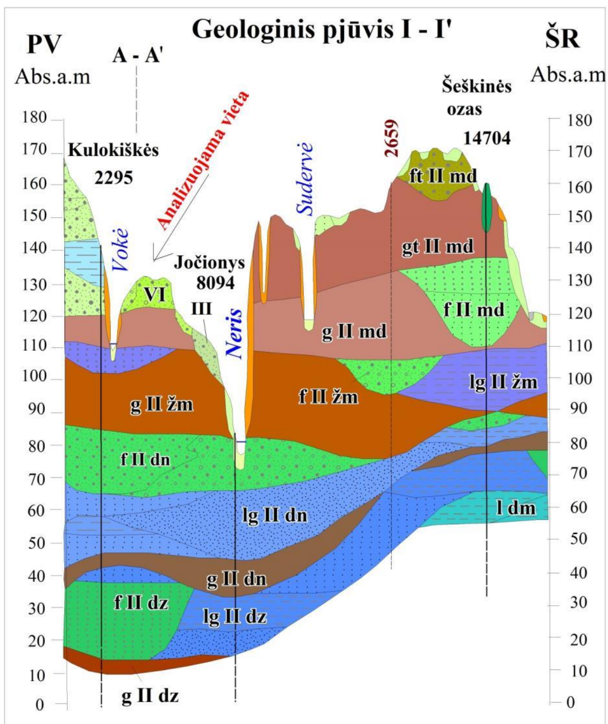
Pav. 4.4.5. Kvartero storymę apibendrinantis geologinis pjūvis I – I' (pagal: Jusienė, 2007.). Pjūvio vieta parodyta 4.4.3 pav., legendą žiūr. 4.4.3a ir 4.4.3b pav.
