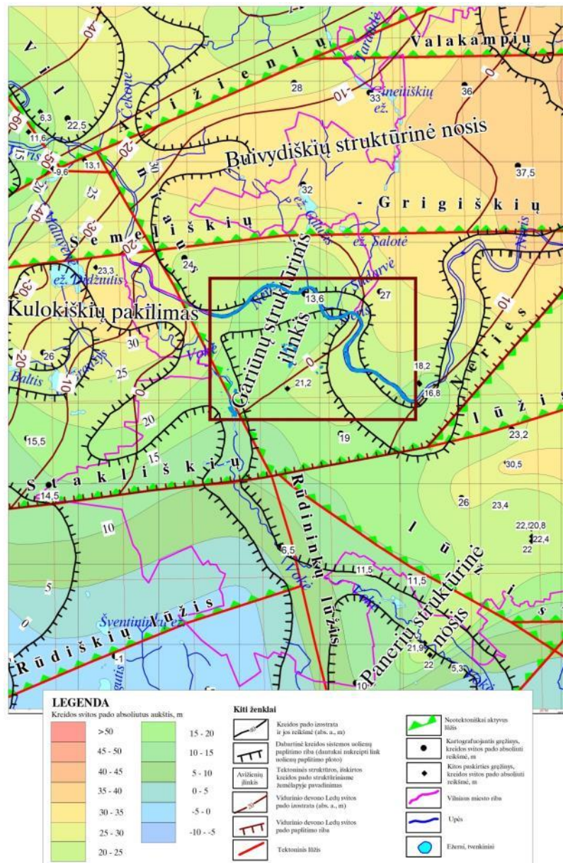
Pav. 4.4.9 pav. Vilniaus miesto tektoninio žemėlapijo (M 1: 25 000) fragmentas. Autoriai: J. Bitinas, J. Čyžienė (Stankevičiūtė ir kt., 2012).
