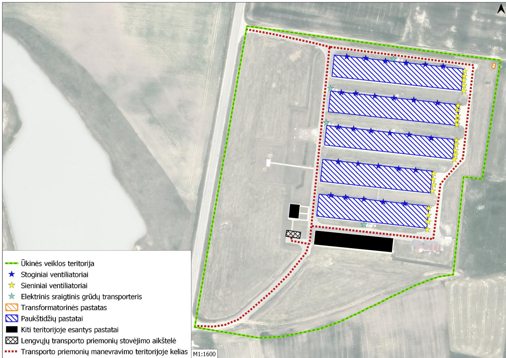
5 pav. Triukšmo šaltinių išsidėstymas ūkinės veiklos teritorijoje
