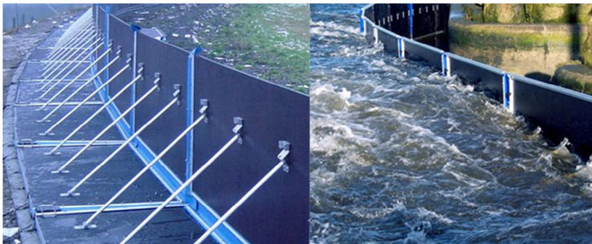
Paveikslas 19. Apsauga nuo potvynių naudojant laikiną surenkamą užtvaramą (šaltinis: http://www.giek.no/en/om_giek/nyheter/unikt_norsk_floemvernsystem_til_usa )
