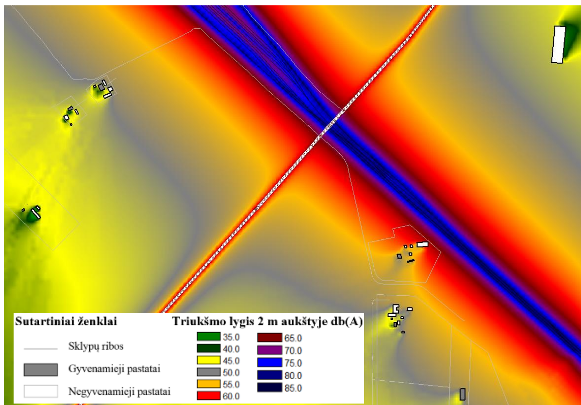
12.9. pav. Prognozuojamas triukšmo lygis nakties metu (Ln)
