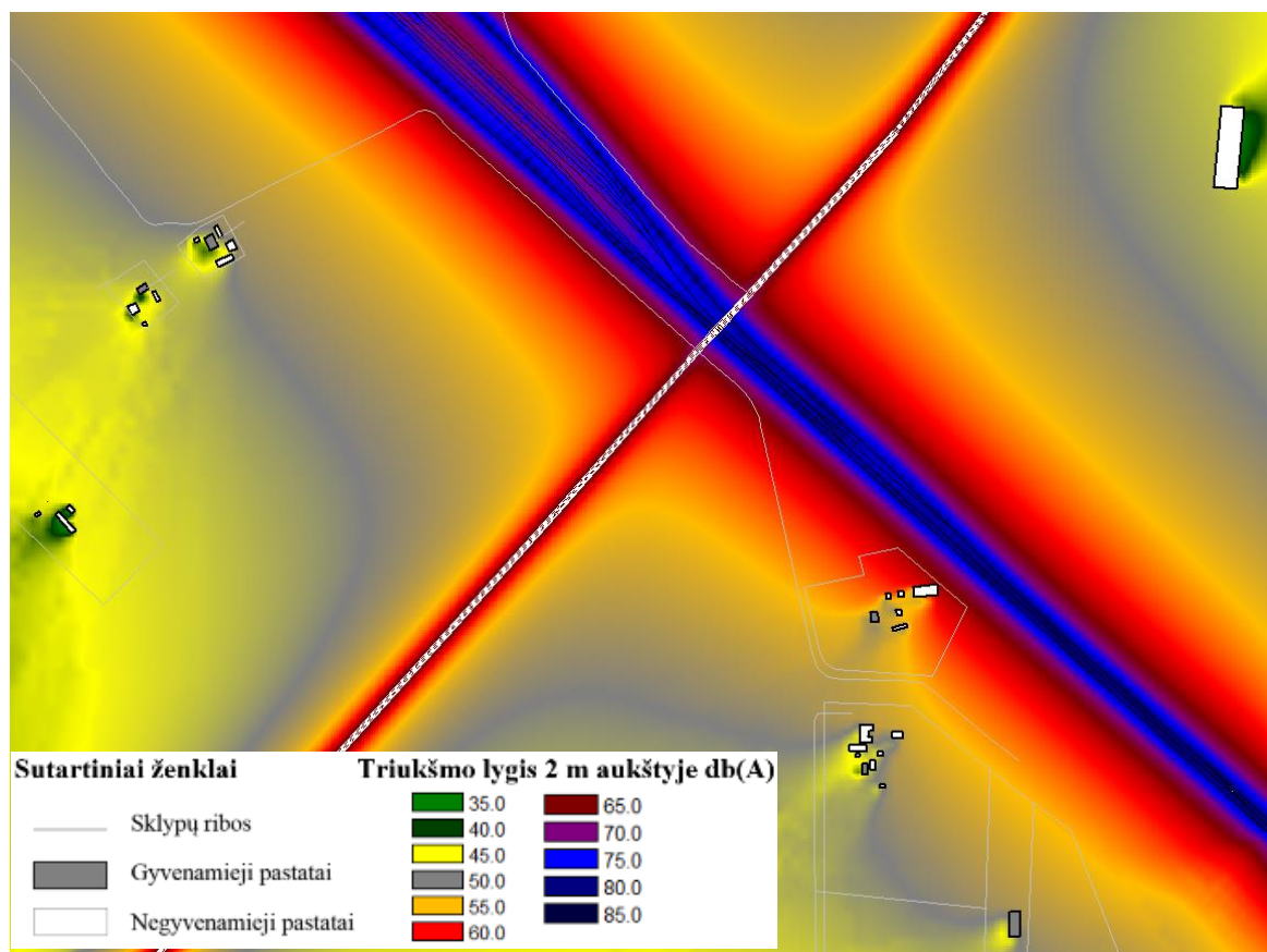
12.8 pav. Prognozuojamas triukšmo lygis vakaro metu (Lv)
