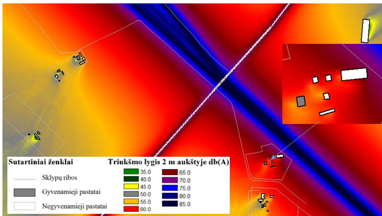
12.11. pav. Prognozuojamas triukšmo lygis dienos, vakaro ir nakties metu (Ldvn)
