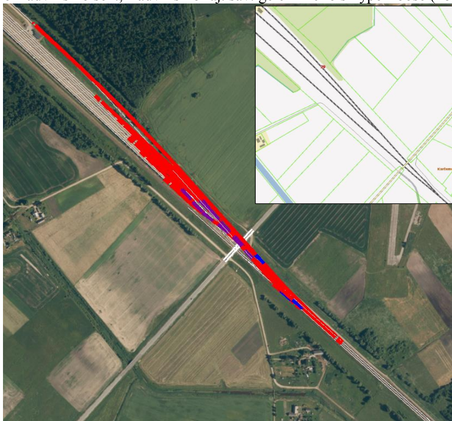
18.2. pav. Radviliškio I atvykimo – išvykimo kelyno kelių ilginimo ir pervažos rekonstrukcijos darbų vieta
