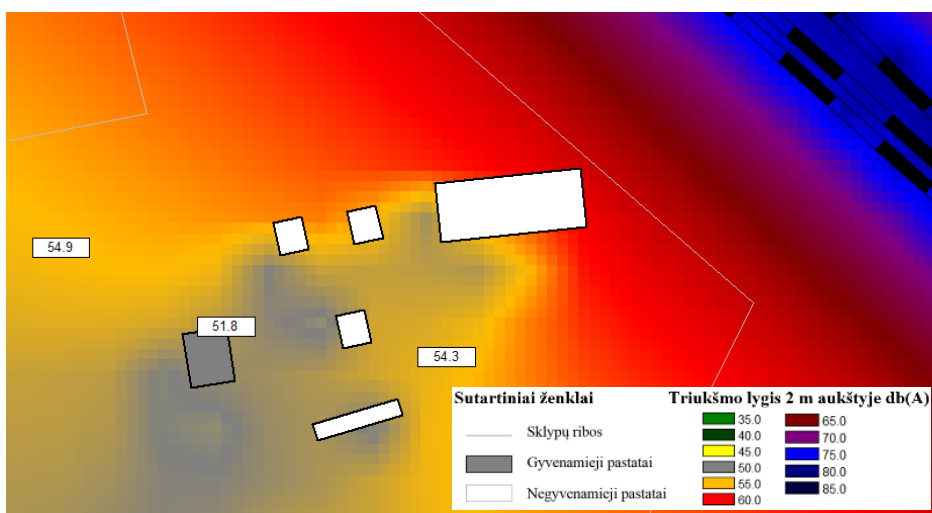
12.10 pav. Prognozuojamas triukšmo ribinių dydžių viršijimas ties gyvenamo pastato gyvenamąja aplinka (40 m.) adresu Pervazos g. 2 (Nr. 2) nakties metu (Ln)
