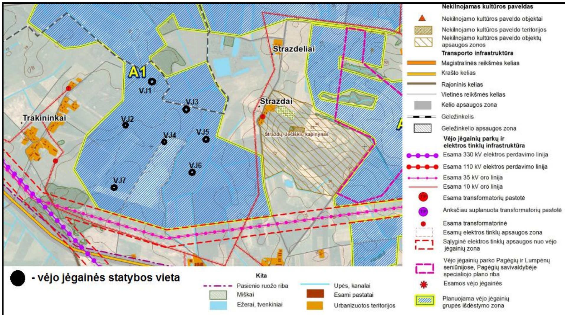
7 pav. Planuojamų vėjo jėgainių statybos vietų situacijos schema Pagėgių sav. vėjo jėgainių parkų išdėstymo specialiojo plano brėžinyje
