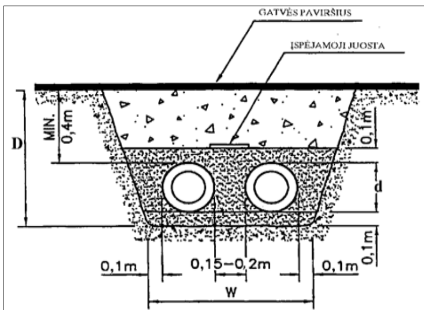
1 pav. Tranšėjų paruošimo ir vamzdžių talpinimo juse matmenys. Šaltinis: Šilumos tiekimo tinklų ir šilumos punktų įrengimo taisyklės
