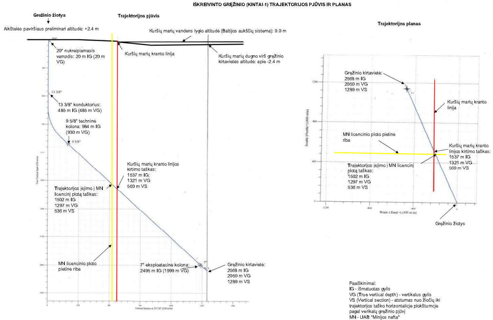
2.1.3 pav. Iškreivinto gręžinio įrengimo schema.
