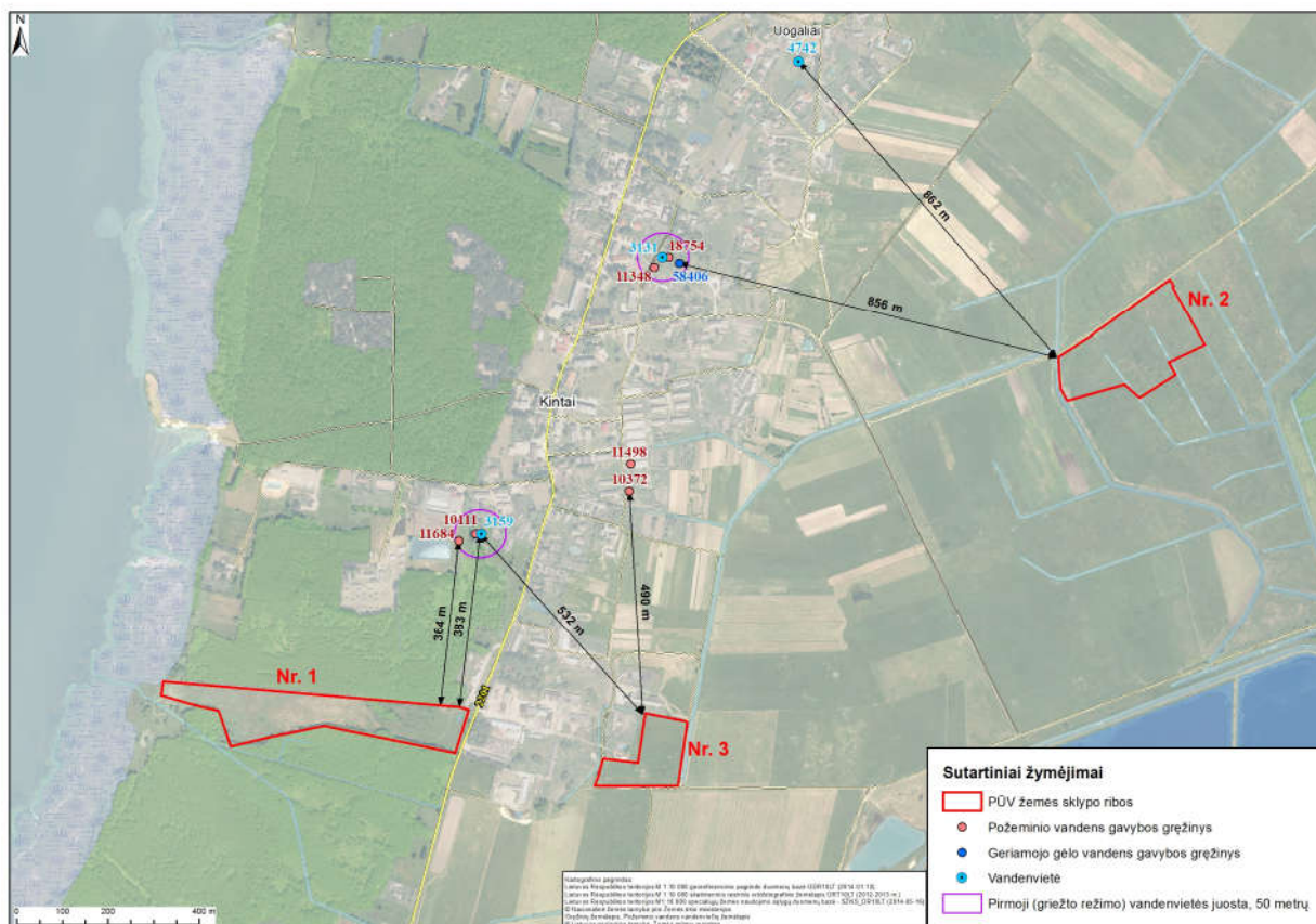
4.1.1 pav. Esamų požeminio vandens vandenviečių išsidėstymas ir apsaugos zona.
