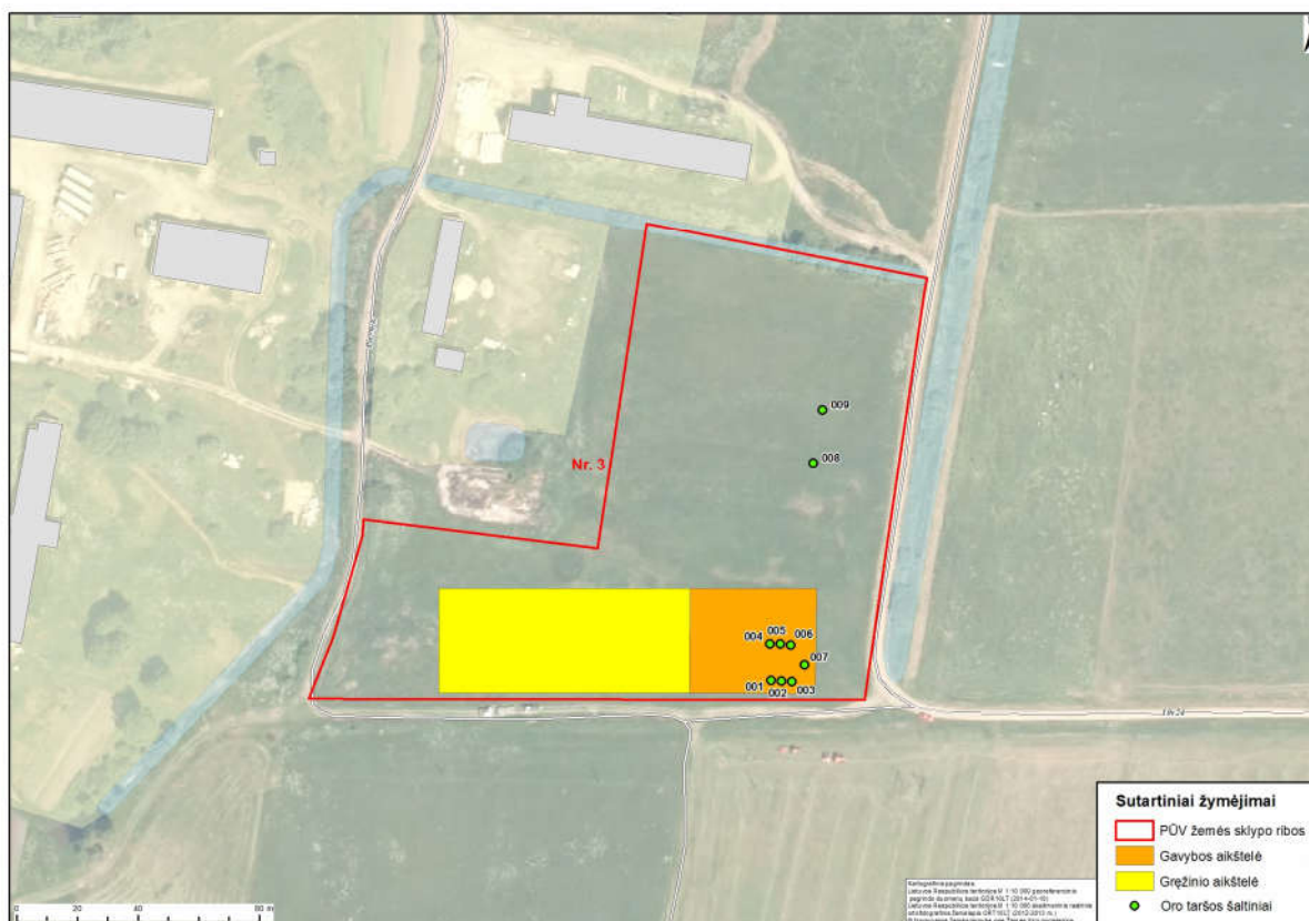
4.2.4 pav. Taršos šaltinių išsidėstymas alternatyvioje Aikštelėje Nr. 3.
