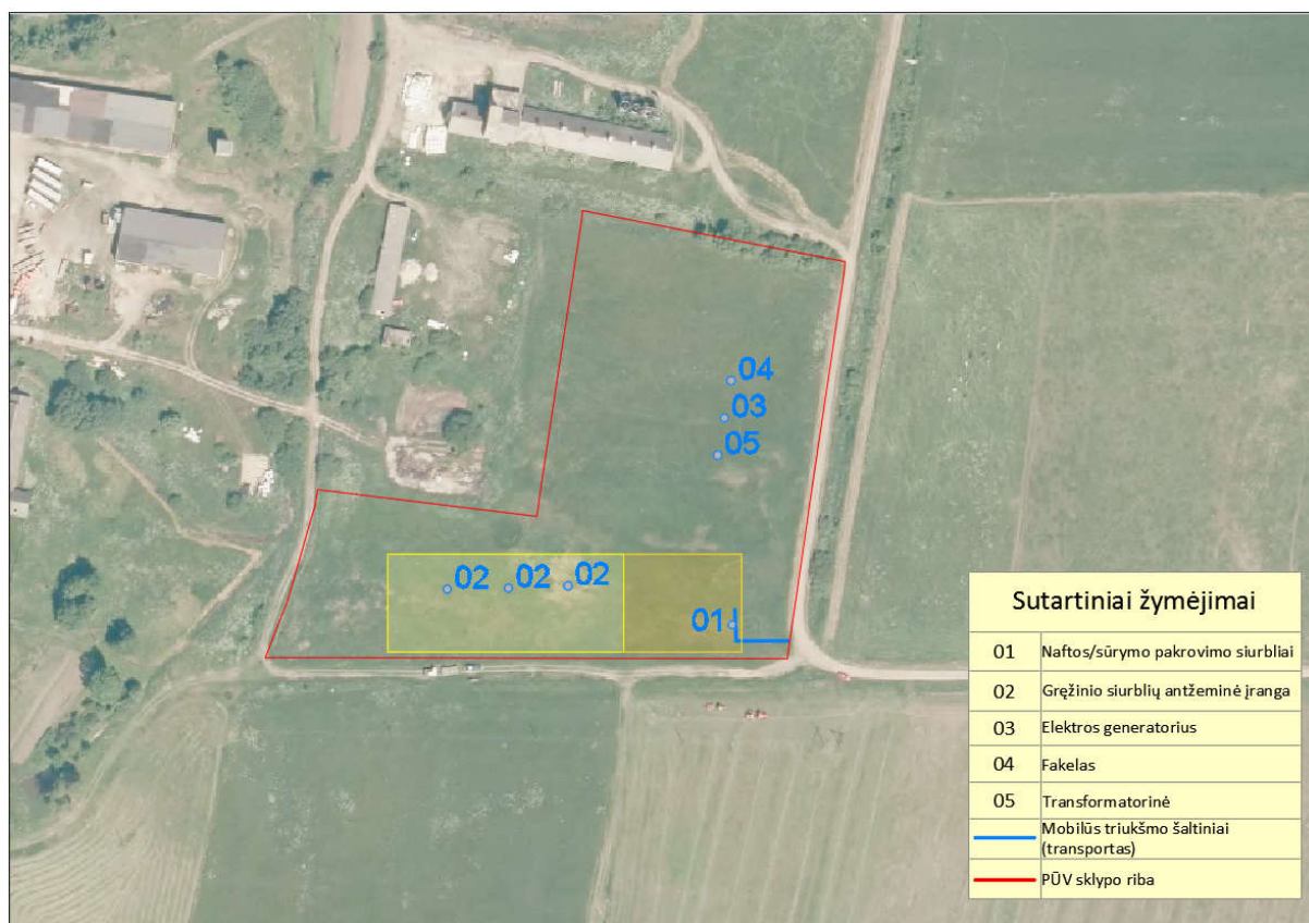
4.9.17 pav. Aikštelės Nr. 3 triukšmo šaltinių schema.
