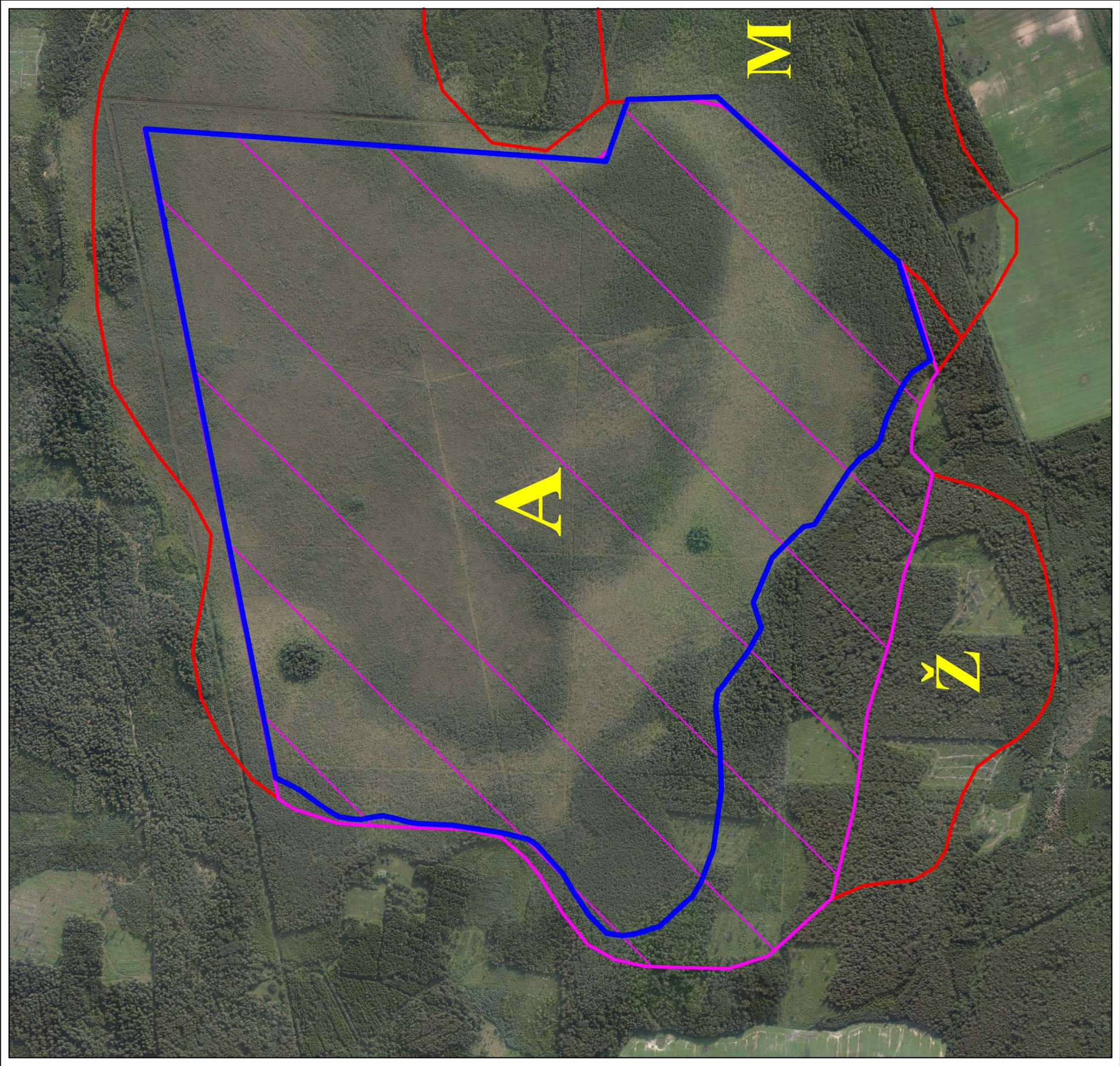
1.3 pav. Juodymo durpių telkinio situacinis ortofotografinis planas M 1:50 000
