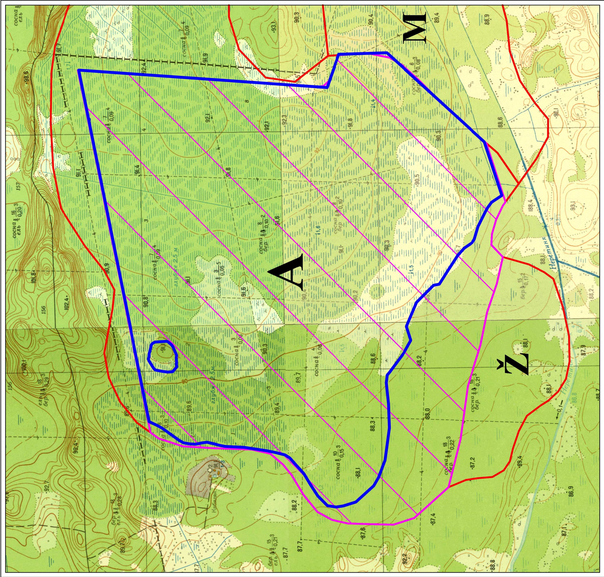
1.2 pav. Juodymo durpių telkinio situacinis planas M 1:50 000 Sutartiniai ženklai
