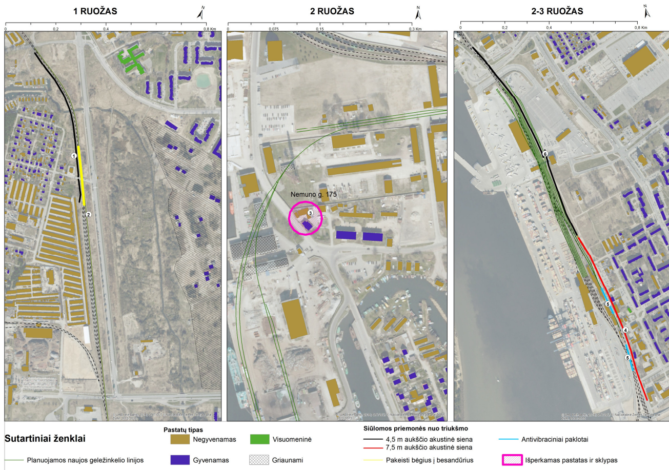
14 pav. Siūlomos aplinkosauginės priemonės nuo triukšmo-vibracijos poveikio 2040 metams
