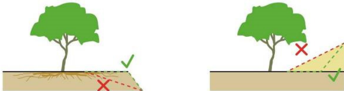
41 pav. Pasirenkant tinkamus techninius sprendinius, formuojant iškasas ir sankasas, galima išsaugoti dalį medžio šaknų
