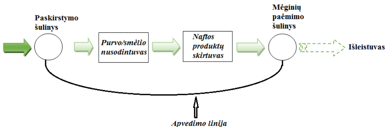
Pav. 1 Siūloma principinė lietaus nuotekų valymo schema
