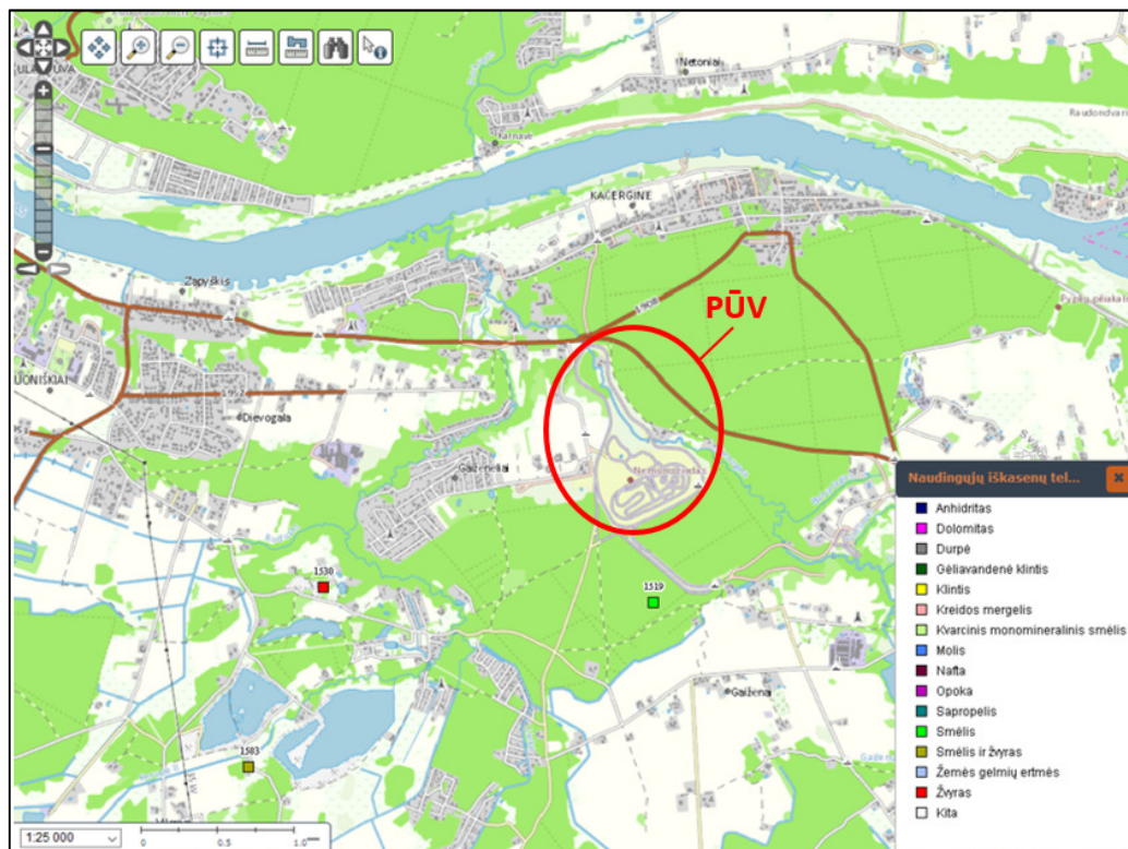
10 pav. Arčiausiai PŪV aptinkami naudingųjų iškasenų telkiniai (ištrauka iš Lietuvos geologijos tarnybos naudingųjų iškasenų telkinių žemėlapių)
