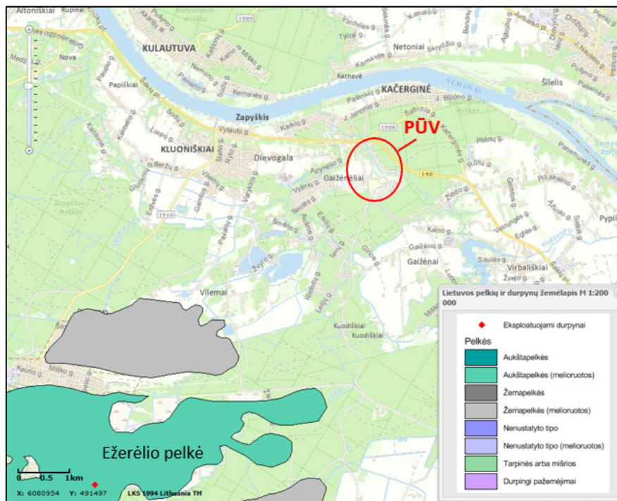
18 pav. Ištrauka iš Lietuvos pelkių ir durpynų žemėlapis (šaltinis: www.lgt.lt)
