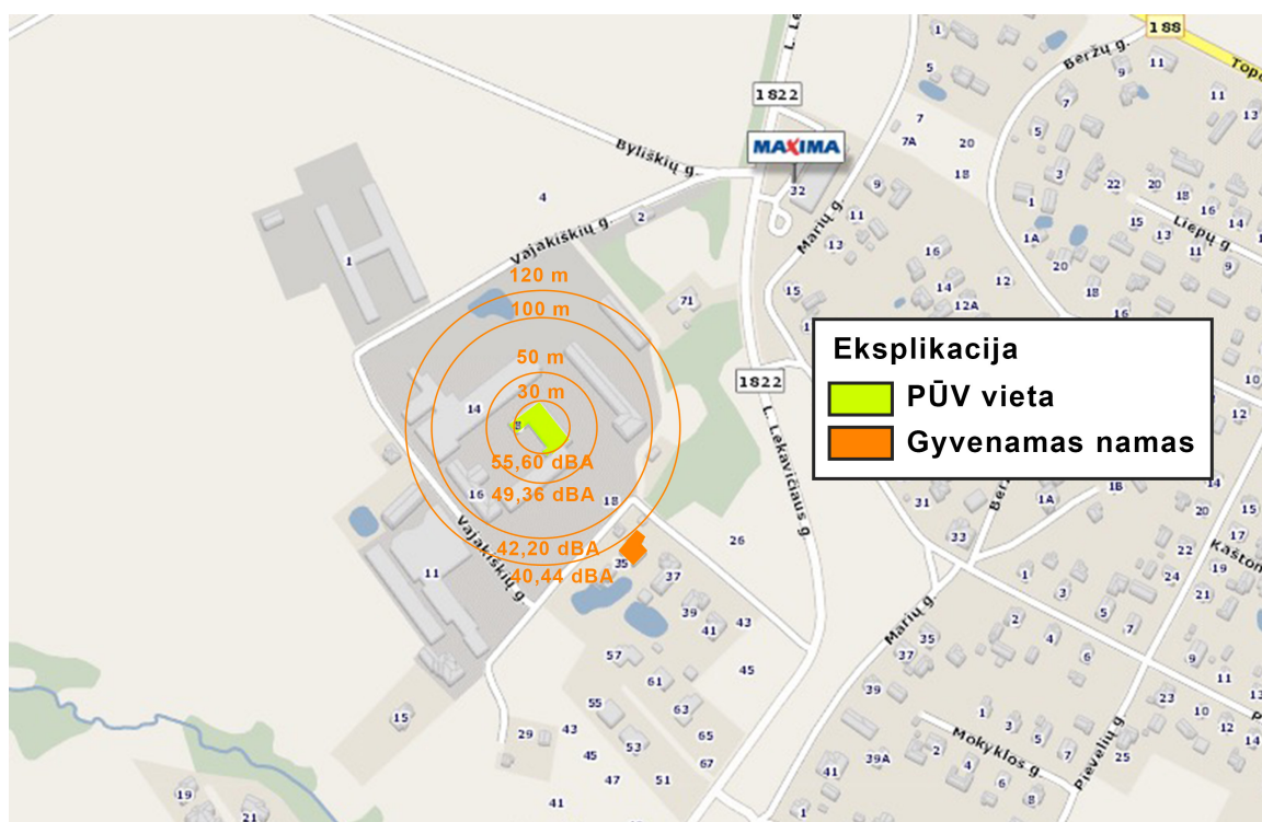
1A paveikslas. Triukšmo lygio sklaidos schema
