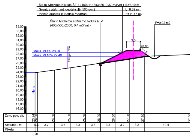
PJŪVIS 22 M1:50
