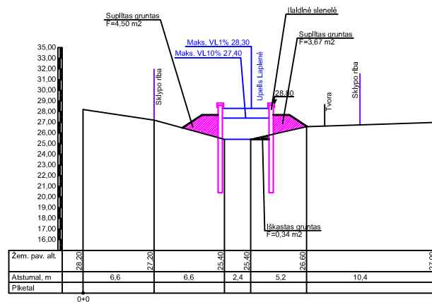
PJŪVIS 24 M1:50
