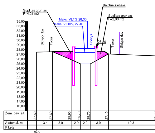
PJŪVIS 27 M1:50
