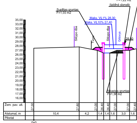
PJŪVIS 28 M1:50
