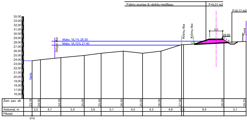
PJŪVIS 17 M1:50
