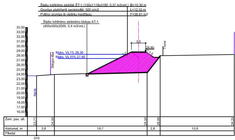
PJŪVIS 21 M1:50
