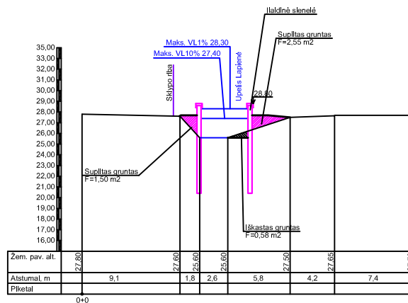
PJŪVIS 22 M1:50
