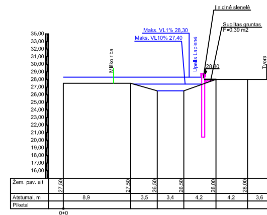
PJŪVIS 26 M1:50
