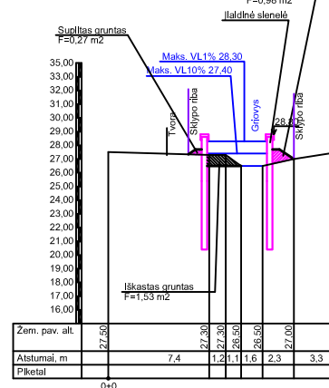
PJŪVIS 29 M1:50
