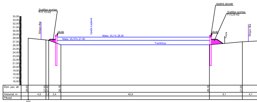
PJŪVIS 27 M1:50
