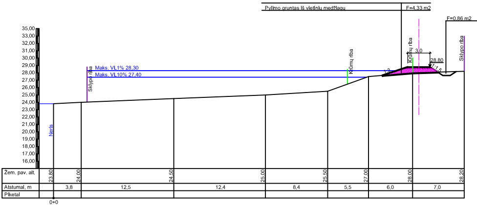
PJŪVIS 16 M1:50
