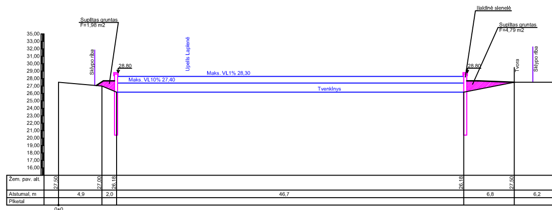
PJŪVIS 29 M1:50
