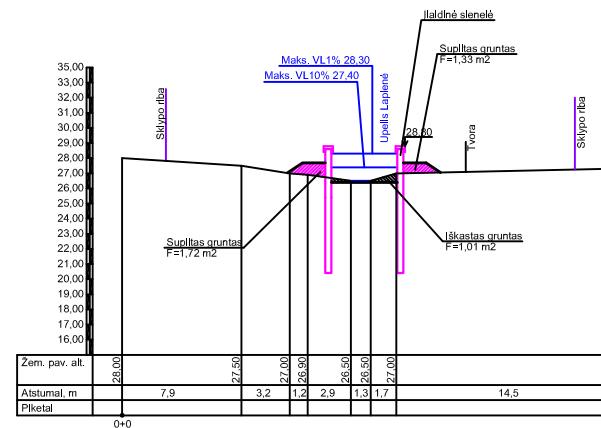
PJŪVIS 25 M1:50
