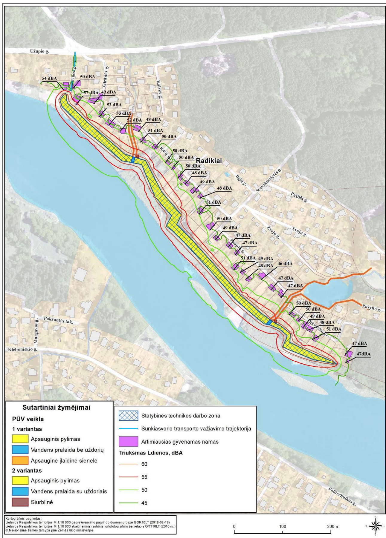
2.11.1 pav. Triukšmo modeliavimo rezultatai.
