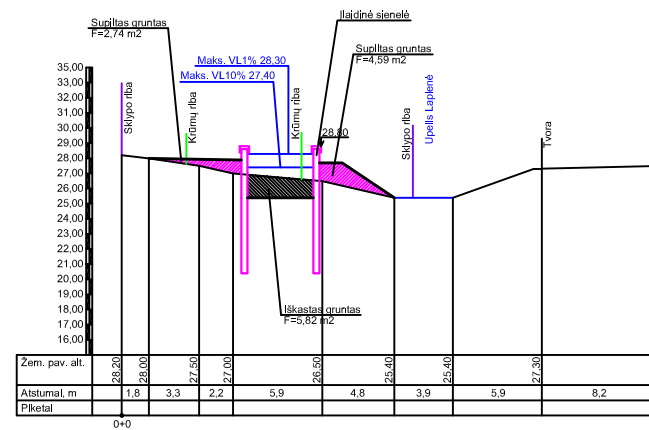
PJŪVIS 23 M1:50
