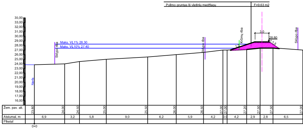
PJŪVIS 17 M1:50
