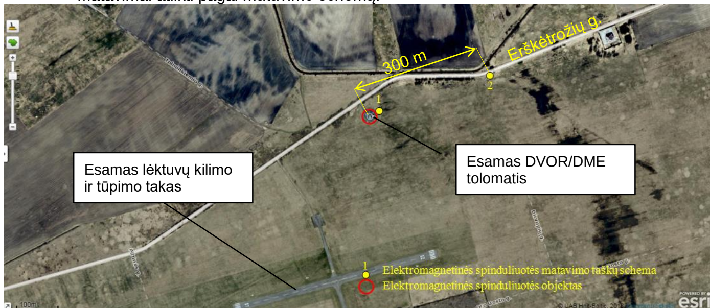
3 pav. Elektromagnetinio lauko matavimo schema
