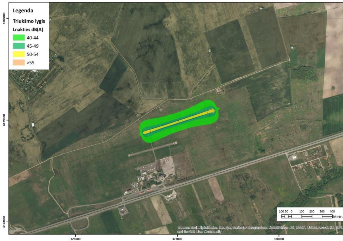
4 pav. Klaipėdos aerodromo pagrindiniu lėktuvų kilimo tūpimo taku, perkeliamu į gruntinio (atsarginio) tako vietą, kylančių ir besileidžiančių lėktuvų prognozuojamas triukšmo lygis ( L_{nakties} triukšmo rodiklis)
