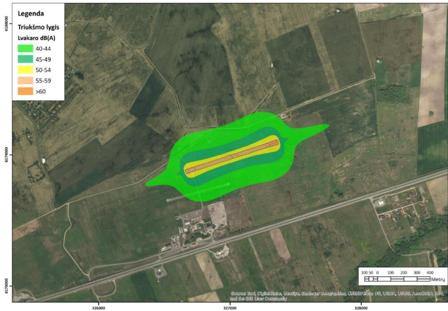
3 pav. Klaipėdos aerodromo pagrindiniu lėktuvų kilimo tūpimo taku, perkeliamu į gruntinio (atsarginio) tako vietą, kylančių ir besileidžiančių lėktuvų prognozuojamas triukšmo lygis (Lvakaro triukšmo rodiklis)
