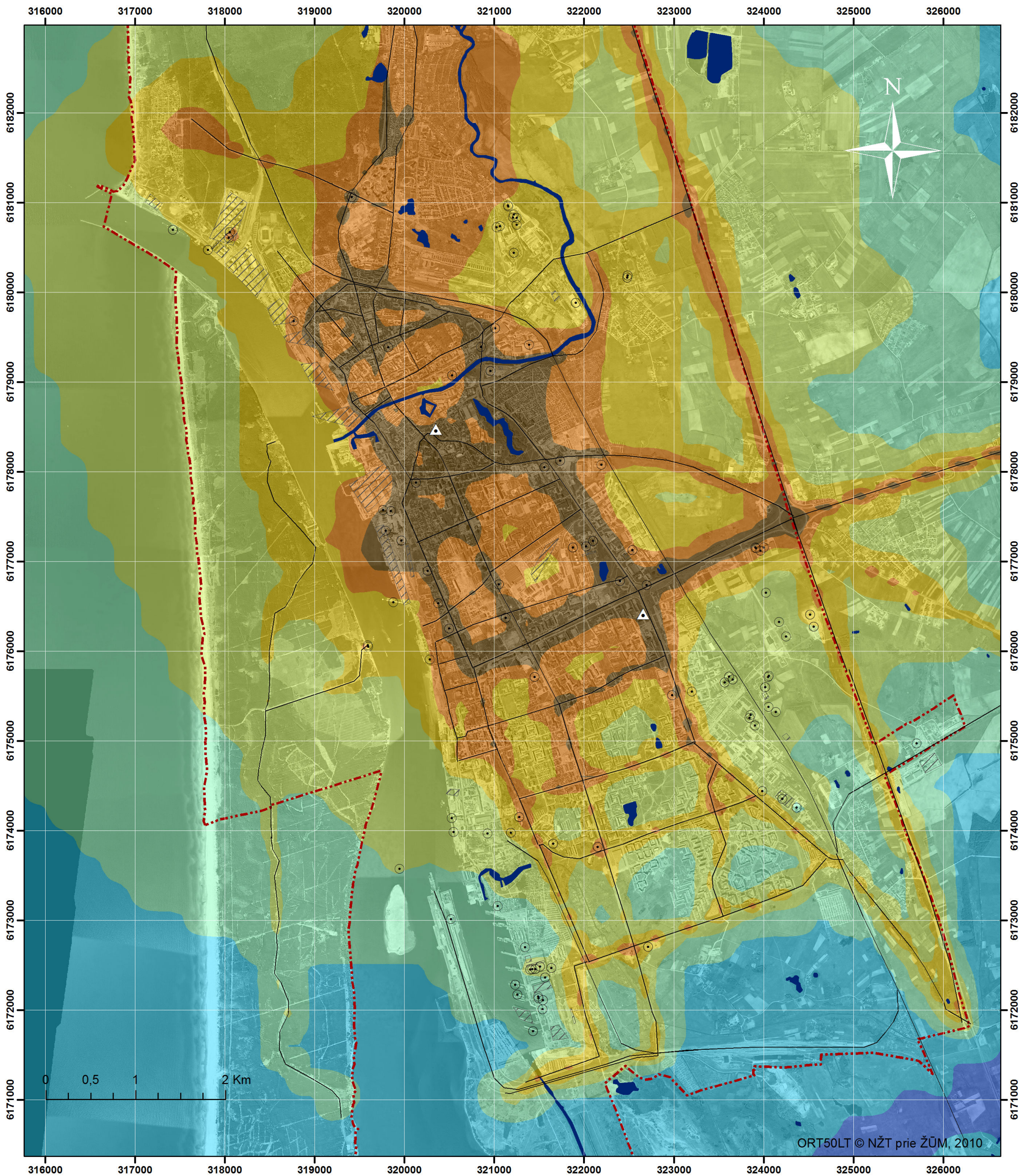
Vidutinė metinė anglies monoksido (CO) koncentracija (mg/m 3 ) aplinkos ore Klaipėdoje 2015 m.
