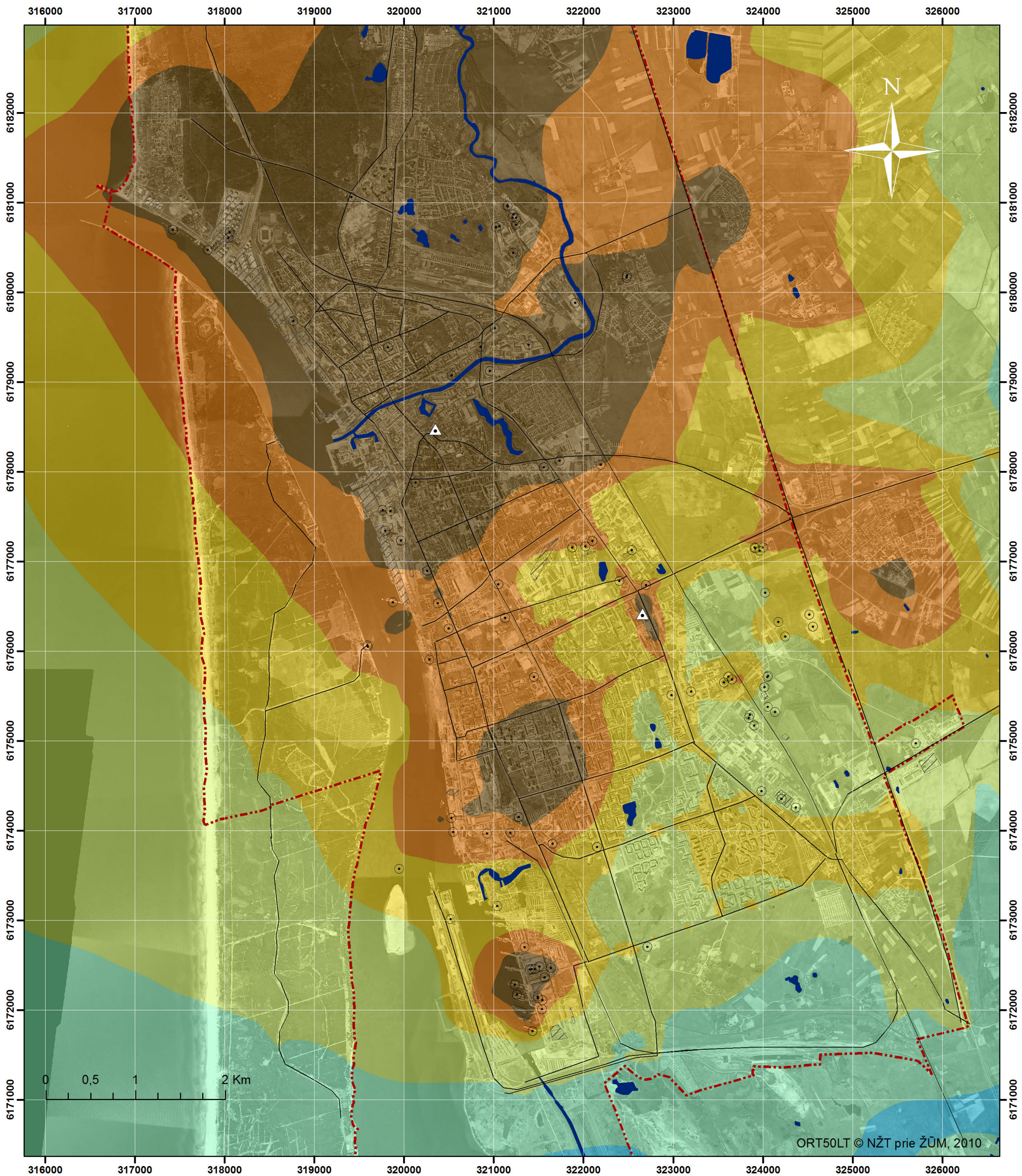
Vidutinė metinė smulkiųjų kietųjų dalelių ( KD_{2,5} ) koncentracija ( \mu\text{g}/\text{m}^3 ) aplinkos ore Klaipėdoje 2015 m. Ribinė vertė 25 \mu\text{g}/\text{m}^3
