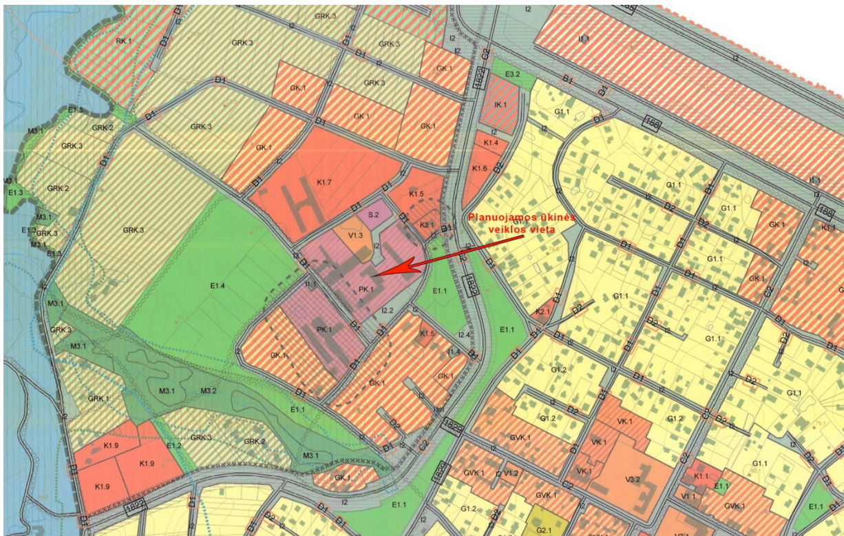
2 paveikslas. Rumšiškių miestelio bendrojo plano teritorijų naudojimo brėžinio fragmentas.
